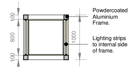
Cube Section A-A 1 : 50
