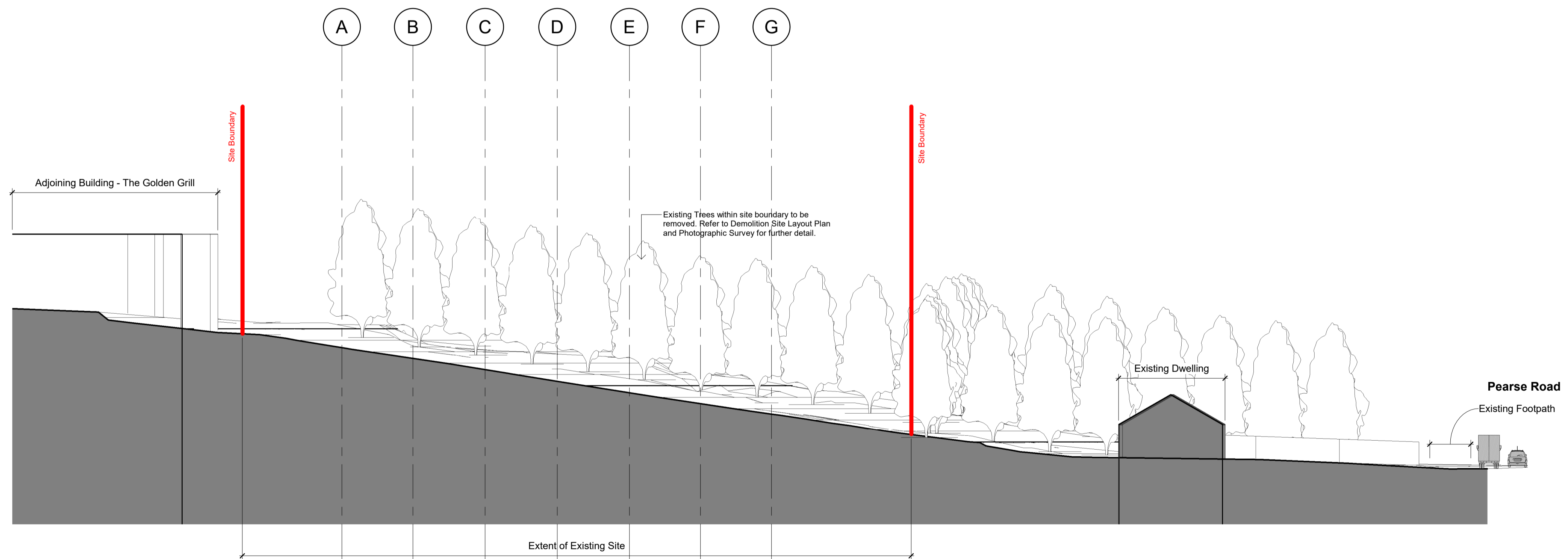
Existing Site Section BB 1 : 250
