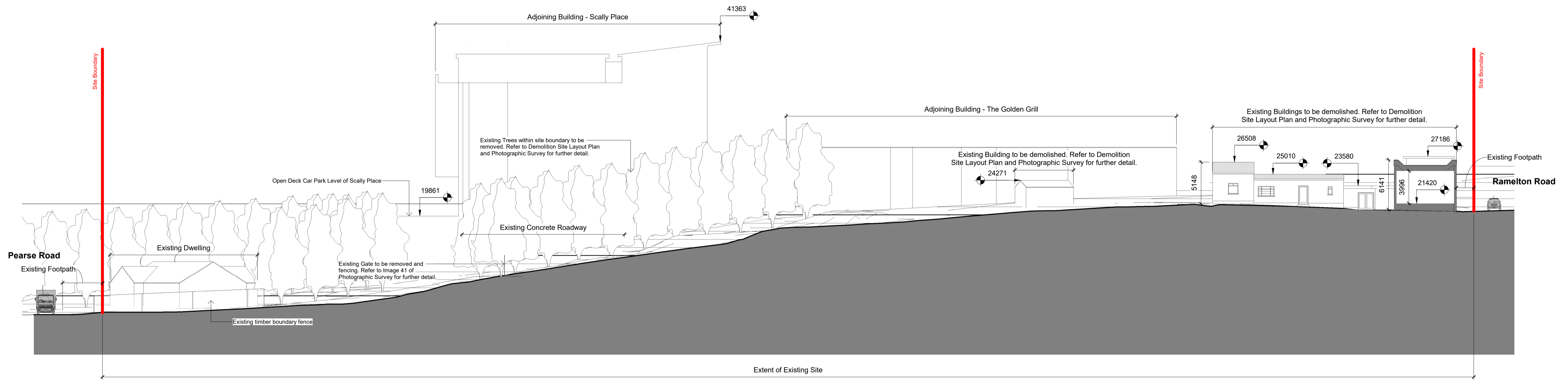
Existing Site Section AA 1 : 250
